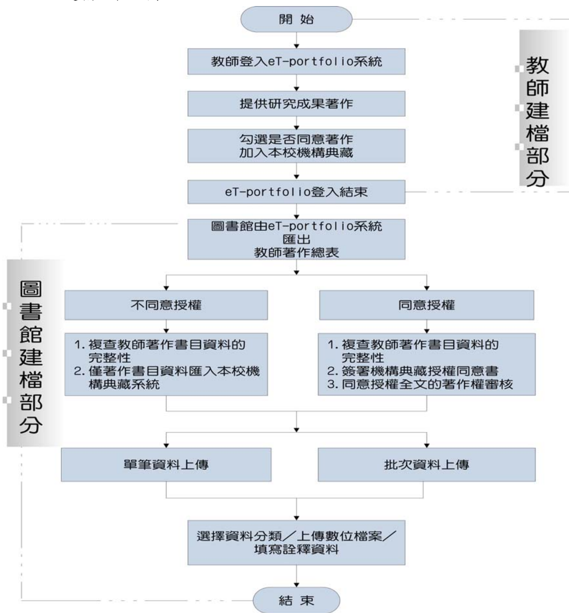
圖4-1 建檔流程圖
