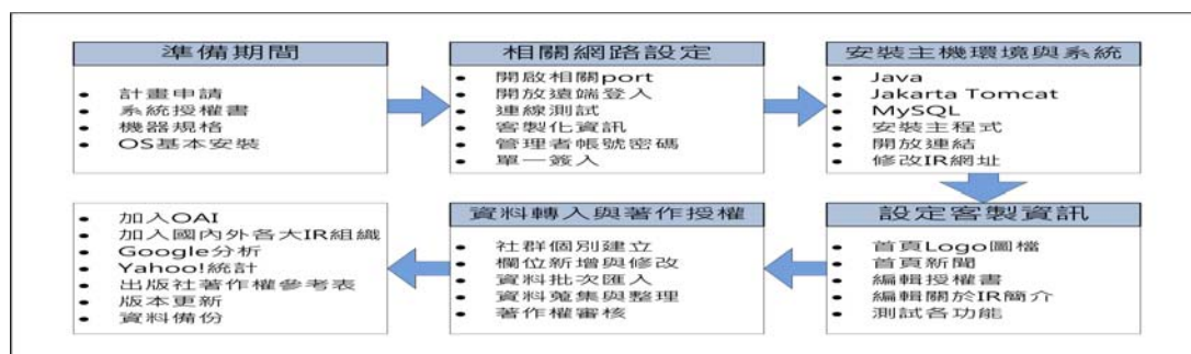
圖 3-1 機構典藏系統執行流程
